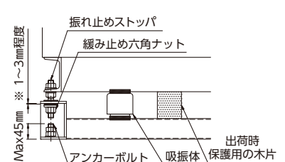
図 4-7 機外防振タイプ
