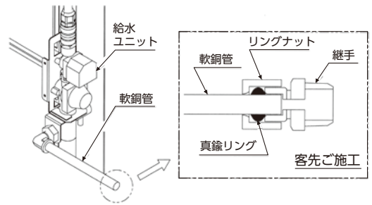
図6-1 気化式加湿器配管施工
