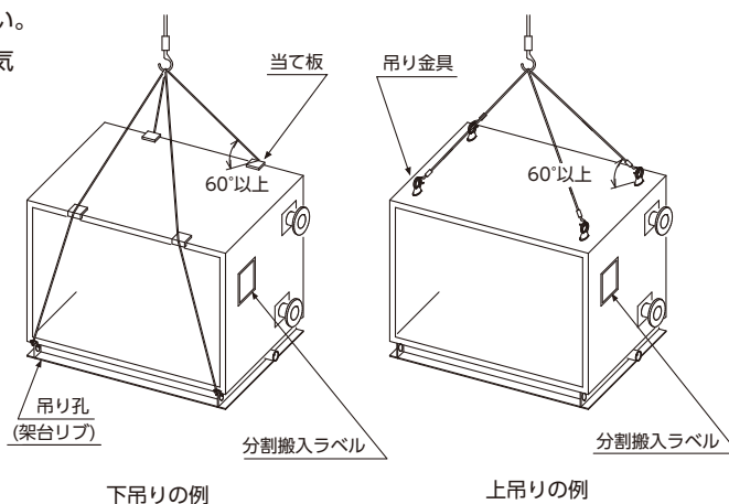
図 3-1 吊り込み例
