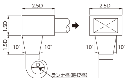
図5-1 ダクト接続距離の例
